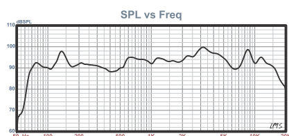
Curva de resposta obtida num box de 25L x 70Hz (1W x 1m).
