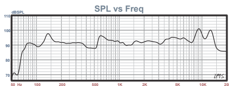
Curva de resposta obtida num box de 15L x 90Hz (1W x 1m).
