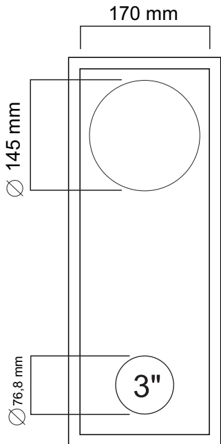
SUGESTÃO 02 - DUTOS REDONDOS
