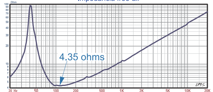
Impedância free-air
